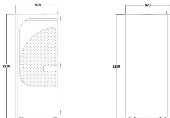
RYSUNEK TECHNICZNY · WYMIARY W MM
