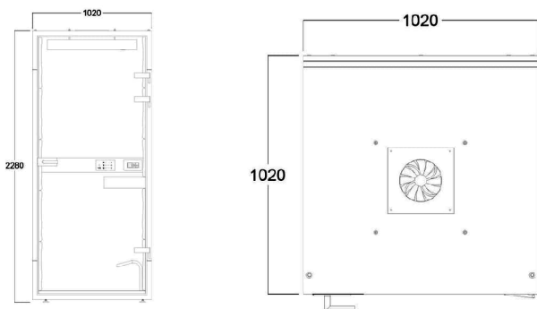
RYSunEK TECHNICZNY · WYMIARY W MM
