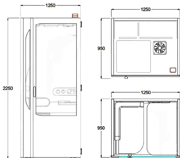
RYSunEK TECHNICZNY · WYMIARY W MM
